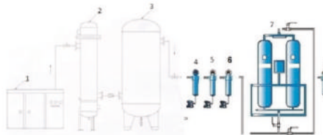
Адсорбционные осушители
